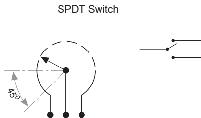
SPDT Switch
